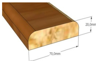
Prierez prahu "D" - na estetické použitie - bez príplatku
