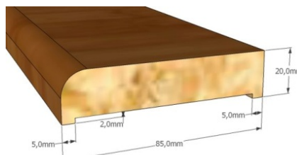
Prierez prahu "U", príplatkový
