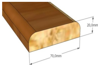
Prierez prahu "D" - na estetické použitie - bez príplatku
